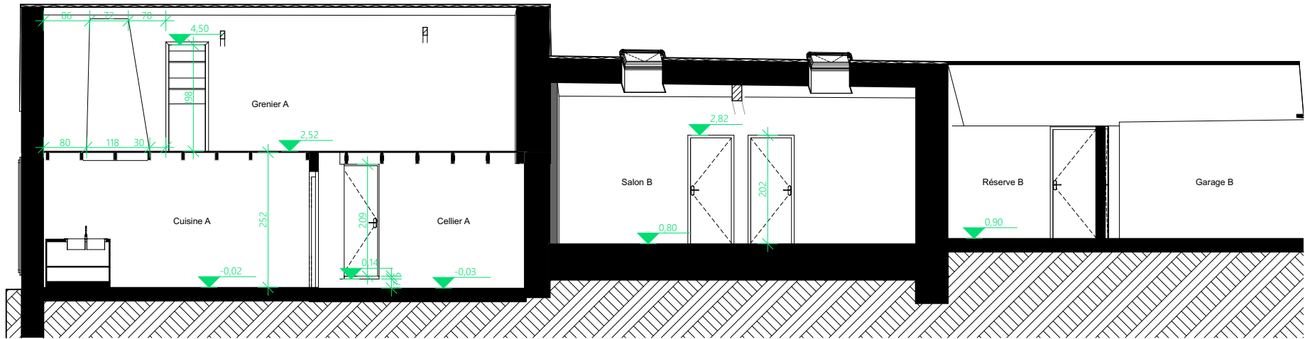
Coupe A3
