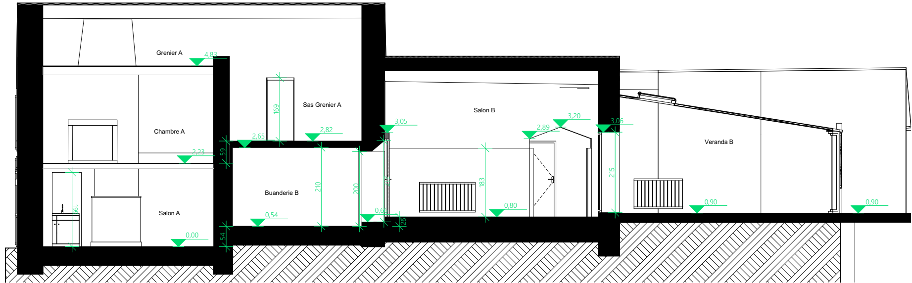
Coupe A2
