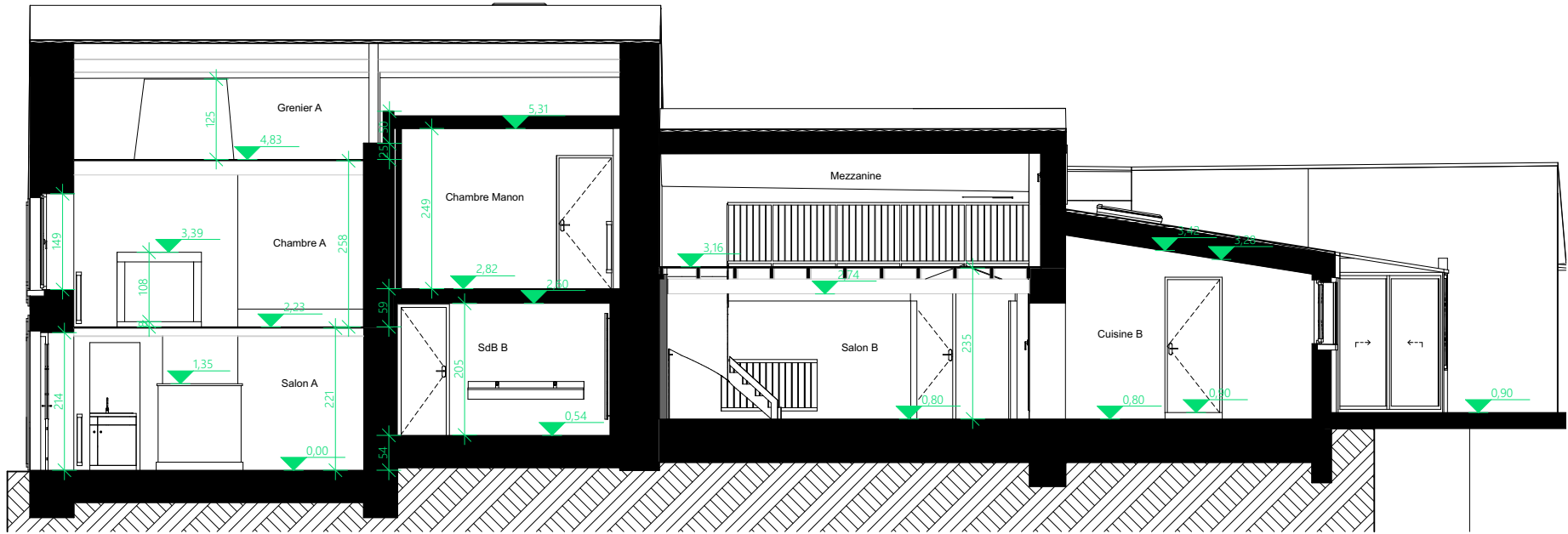
Coupe A1
