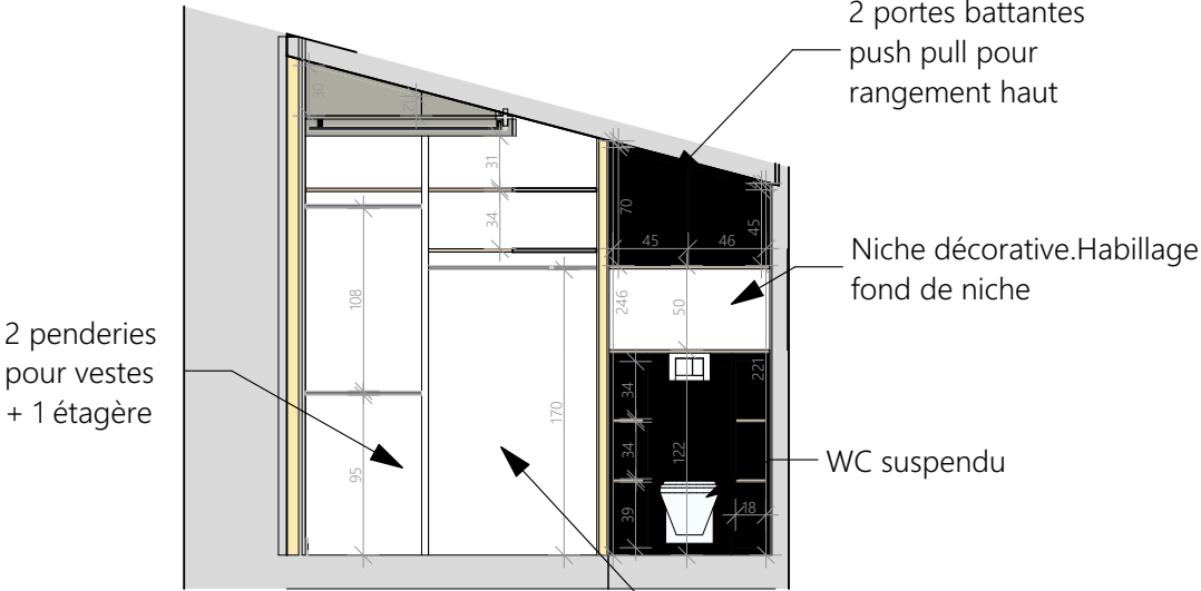
Coupe CC
