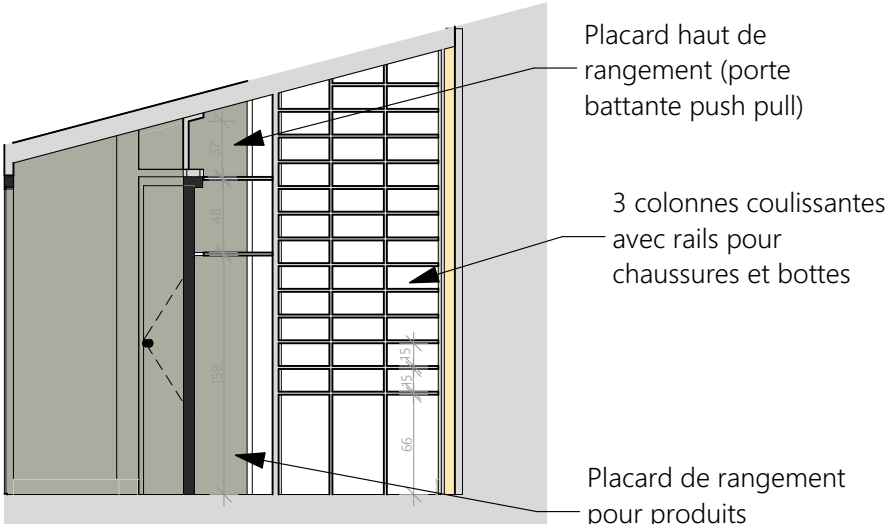
Coupe EE
