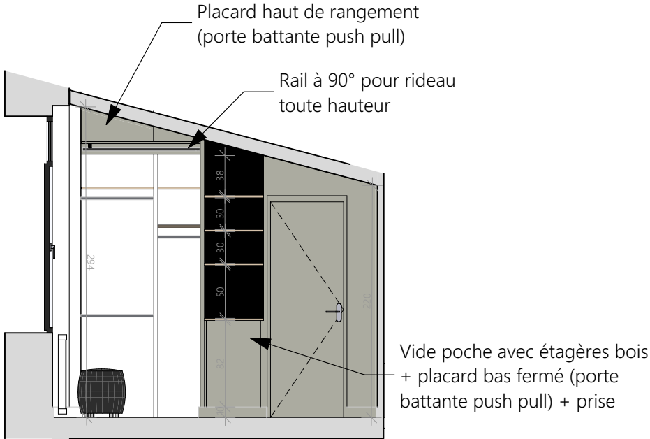
Coupe DD
