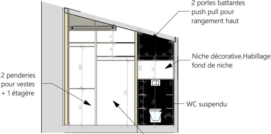
Coupe CC
