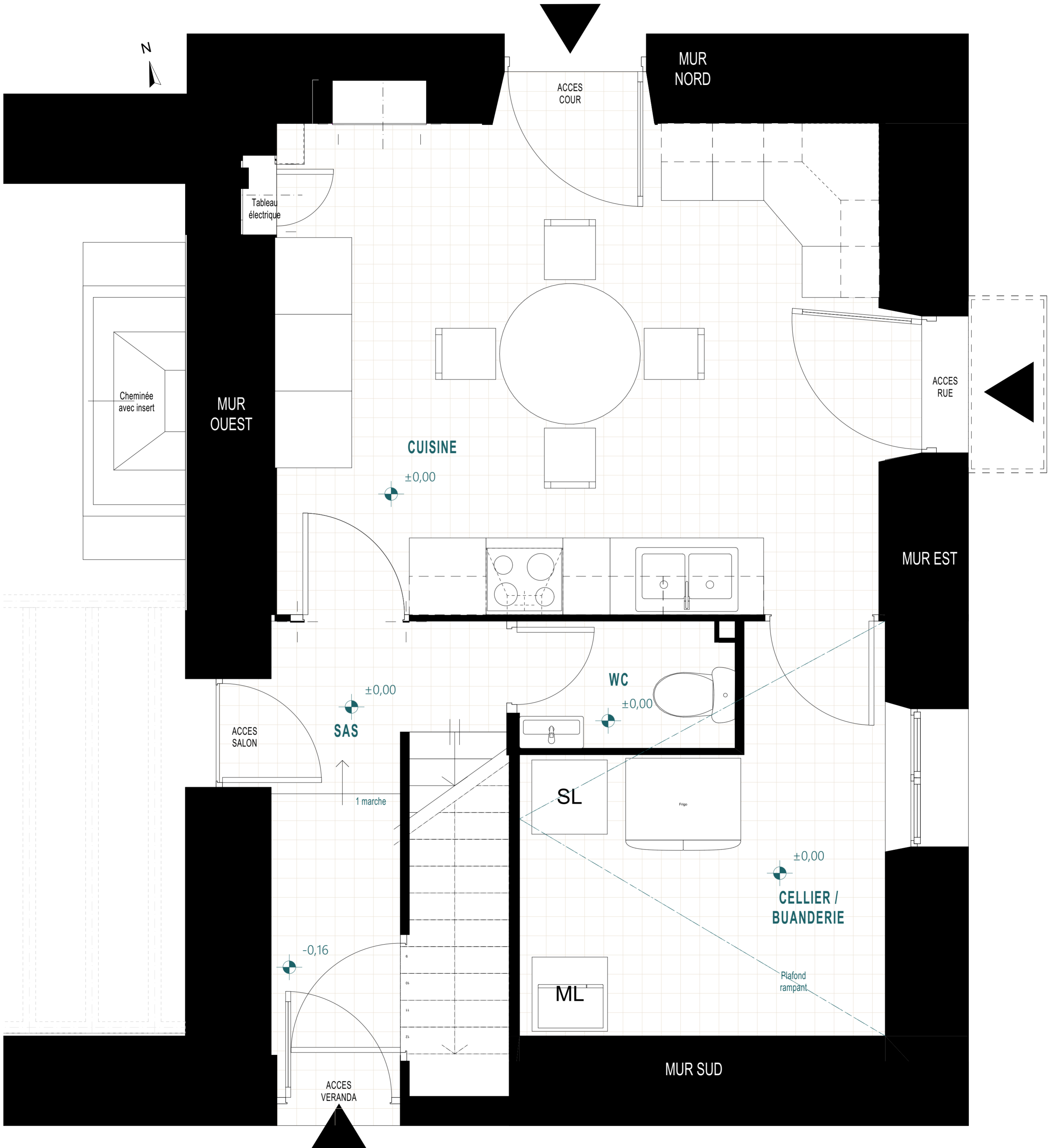
Plan Rdc Existant - 20ème:20
