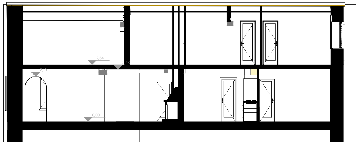
Coupe BB Existant 1:100
