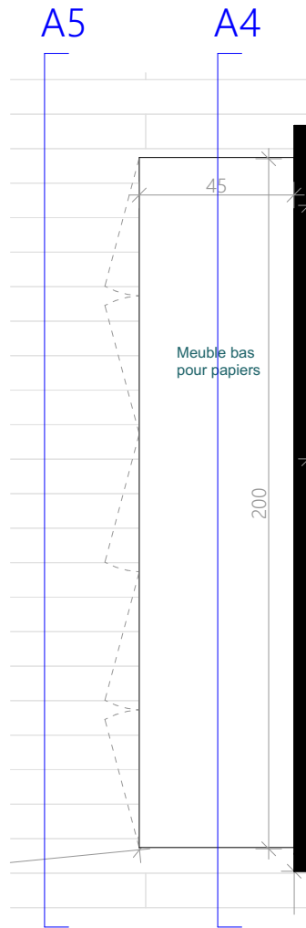
Meuble papiers - Plan - 20ème
