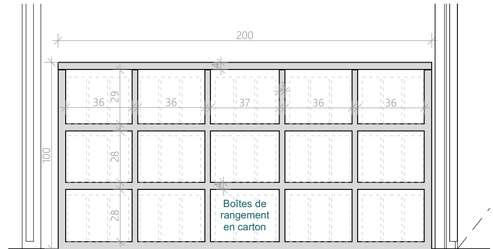
Meuble papiers - Coupe A4 - 20ème
